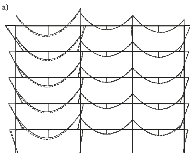
Рисунок 3 – Эпюры изгибающих моментов в раме Р-3: а) при расчетной нагрузке; б) при нагрузке, предшествующей разрушению
